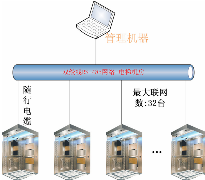
RS-485网络图
